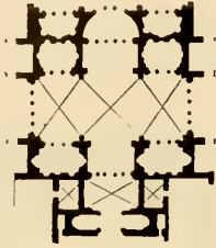
Fig. 111 — Planta di una sala della terme di Nerone a Roma (a. 228) (Dal Palladio «Le terme di Roma»)
